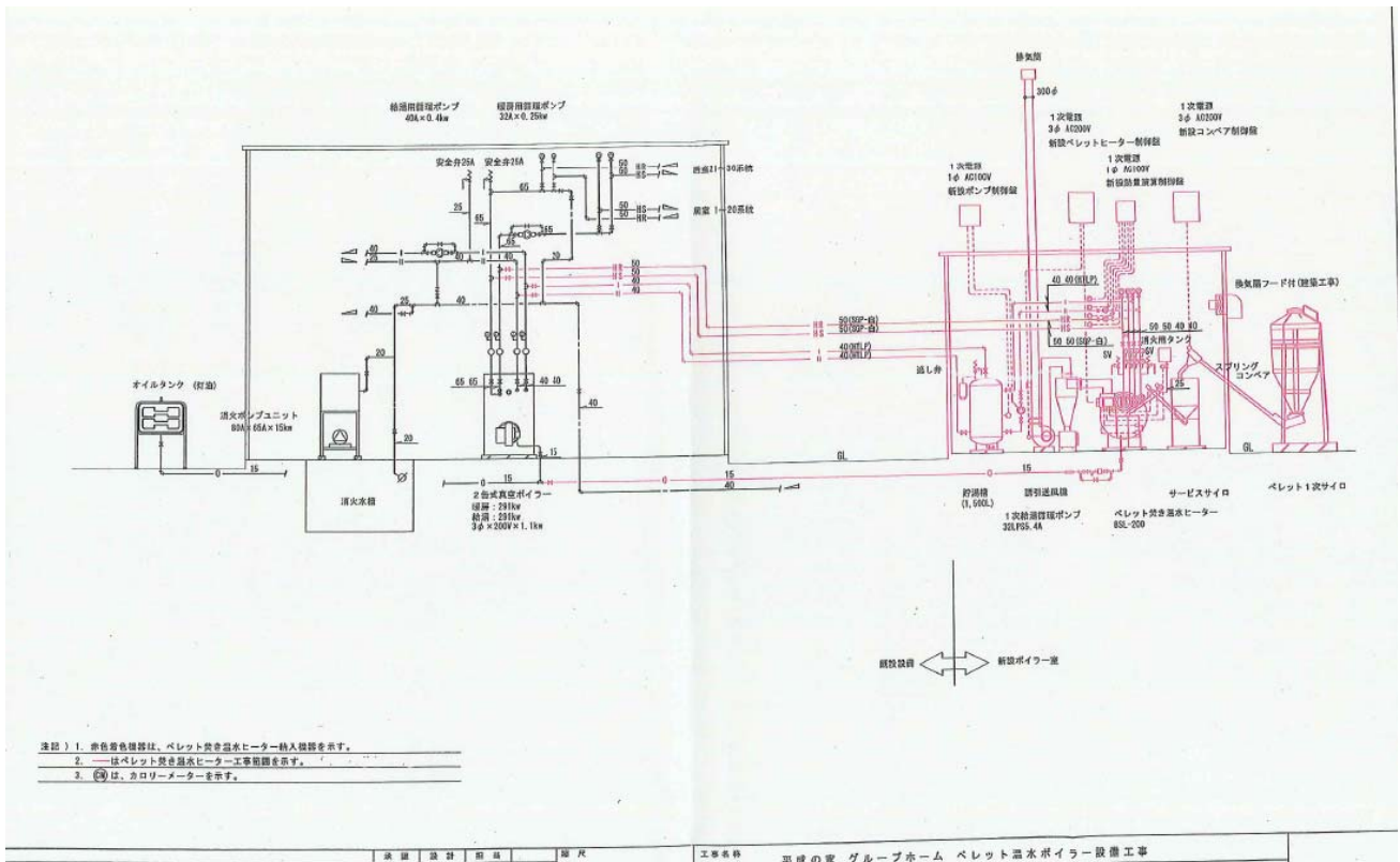
図3 実施後設備配置図 (配管図)
