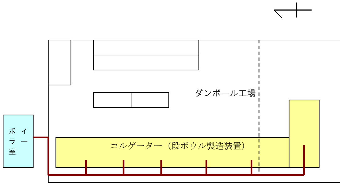
久門紙器工業株式会社における蒸気の配管概略図
