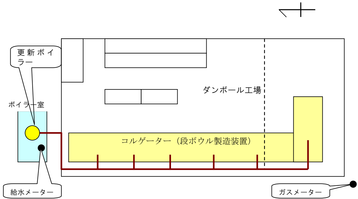
久門紙器工業株式会社における蒸気の配管概略図と測定機器
