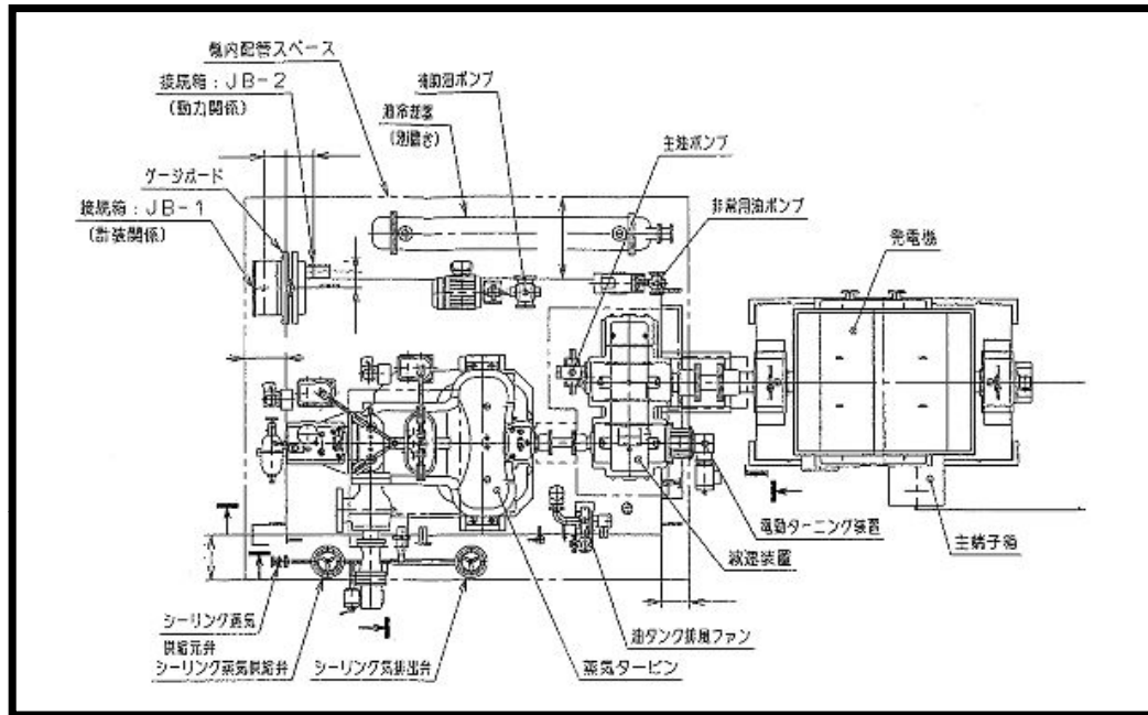
・蒸気タービン発電機 図面
