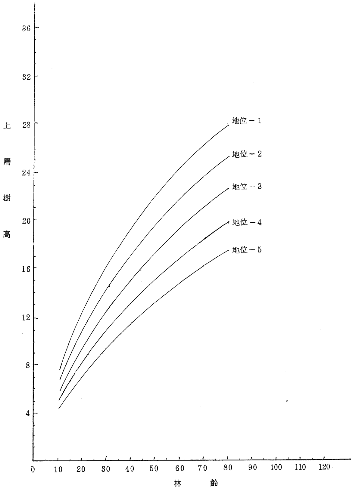
ヒノキ、地位別上層樹高曲線図
