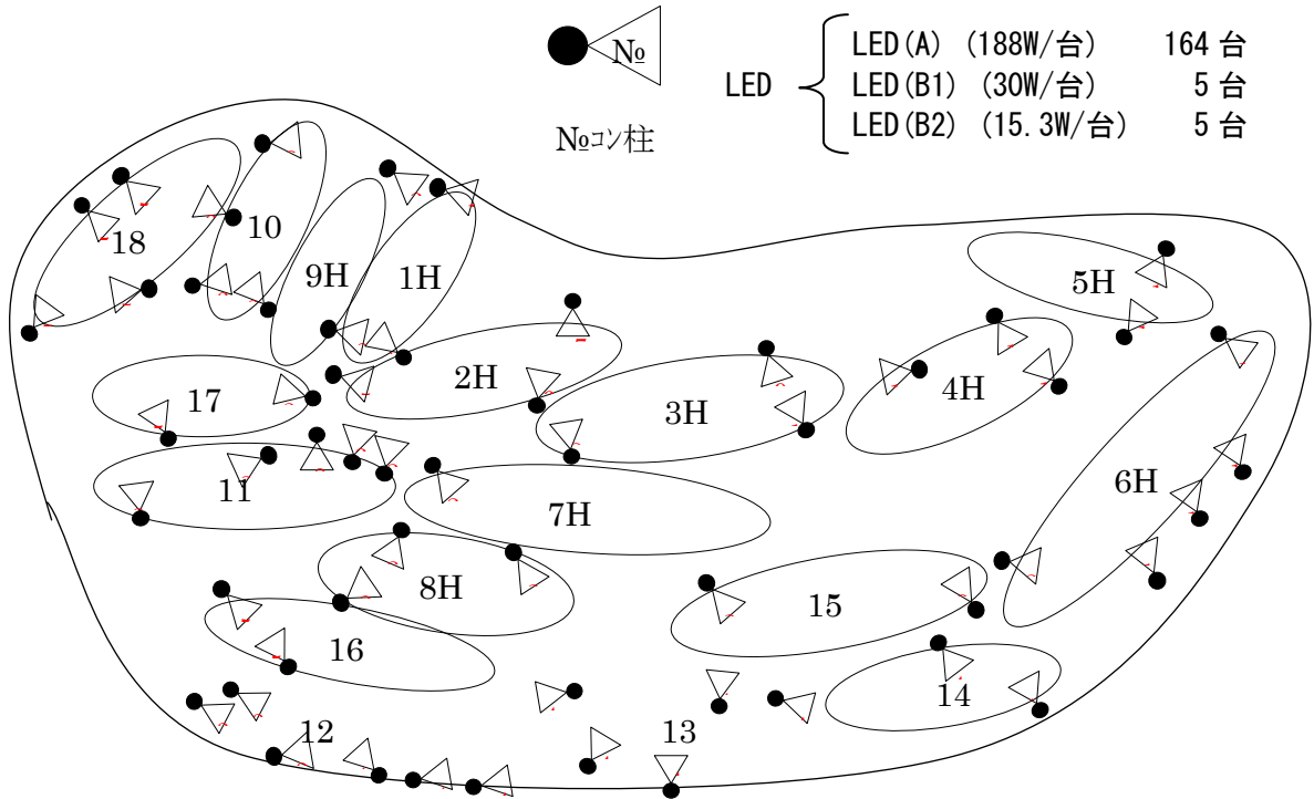
コース内夜間照明設備配置図
